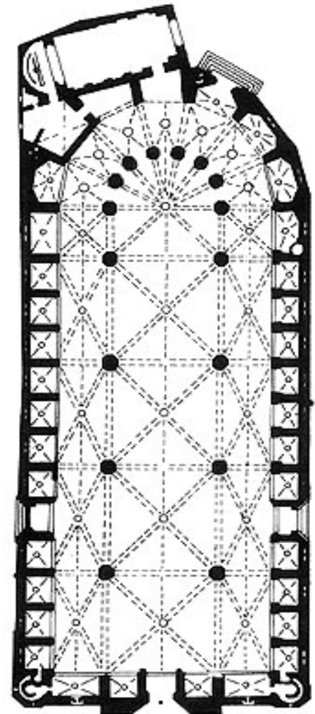
Planta de l'església. Santa Maria del Mar.
