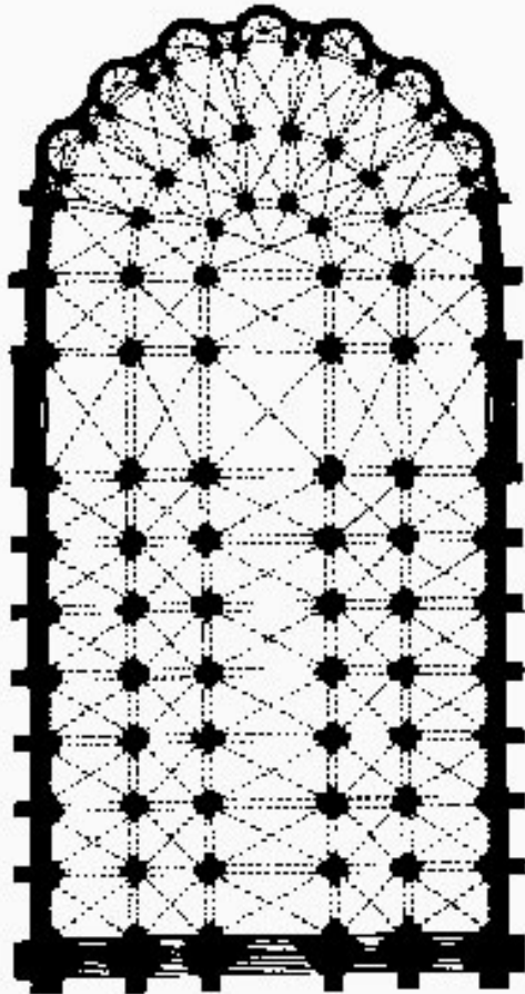
Planta de la catedral; s. XIII. Toledo.
