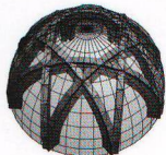
De arcos entrecruzados
